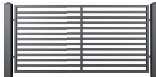
AW.10.111 (blacha pełna, blacha perforowana: Qg 5-8, Qg 10-30, v 5-8)
