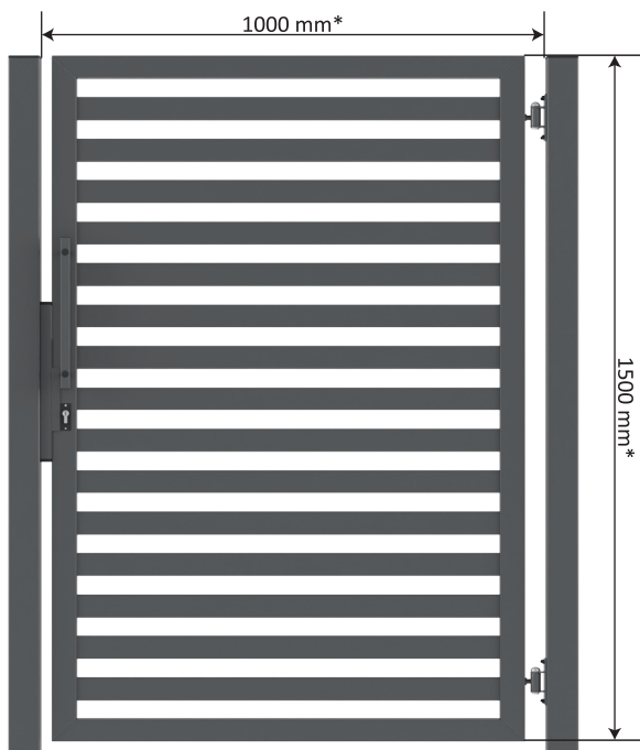
Furtka standartowa
